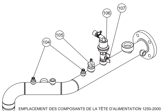
EMPLACEMENT DES COMPOSANTS DE LA TÊTE D'ALIMENTATION 1250-2000
