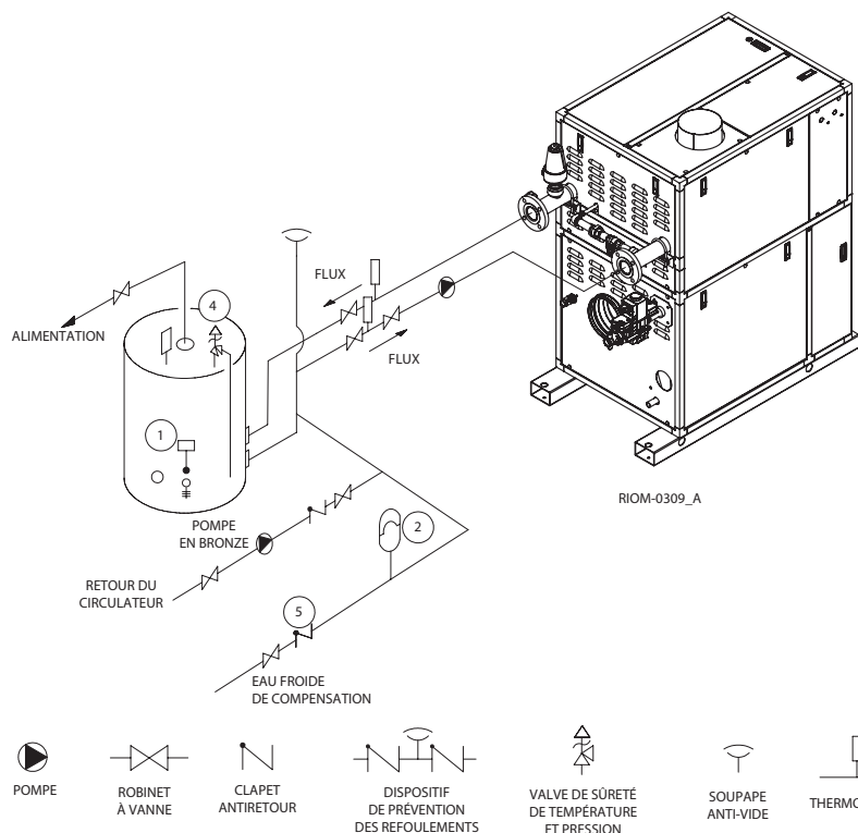
Figure 15 – Chaudière multiple typique avec tuyauterie de réservoir de stockage direct
