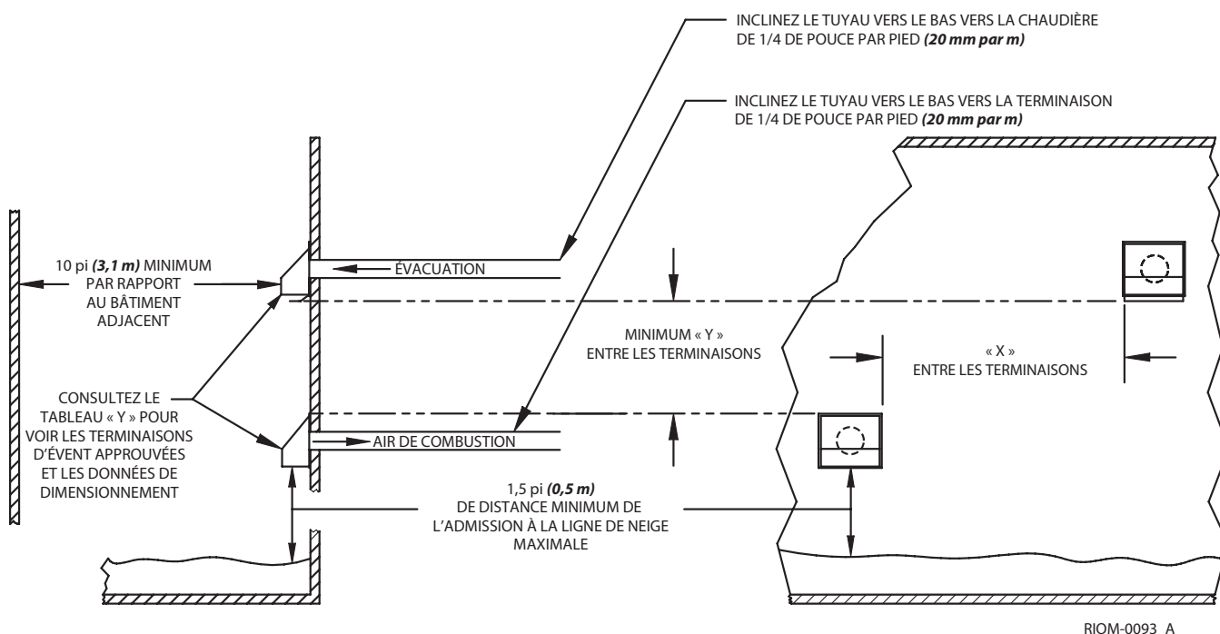
Figure 2 – Prise d'air et ventilation horizontale pour un système à évacuation directe simple
