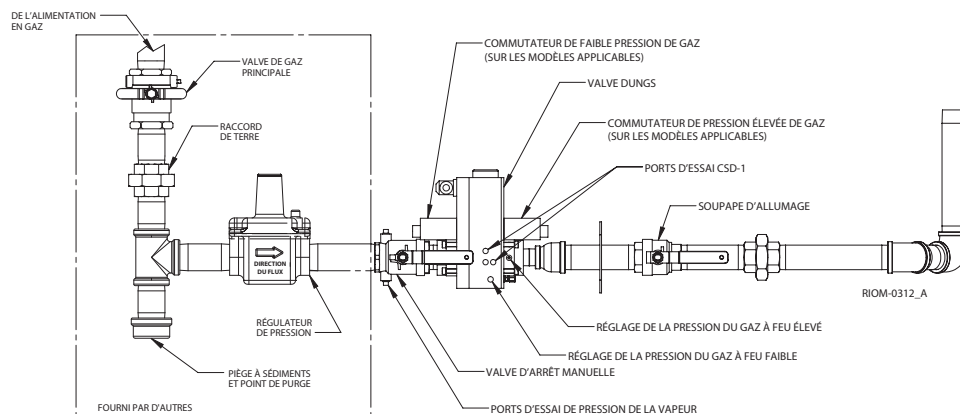
Figure 17 – Tuyauterie d'alimentation en gaz
