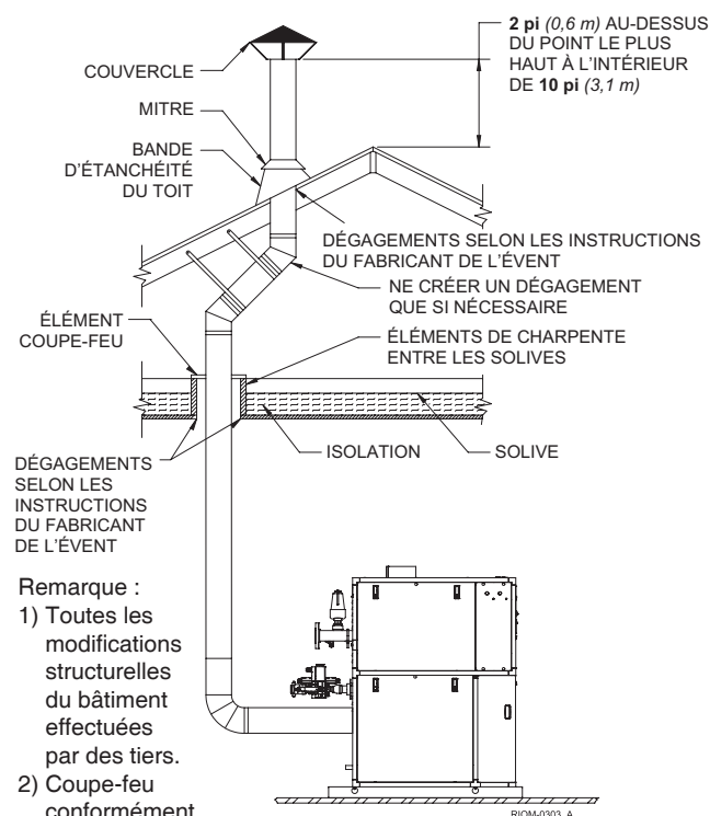
Figure 8 – Ventilation verticale avec un système de cheminée en métal
