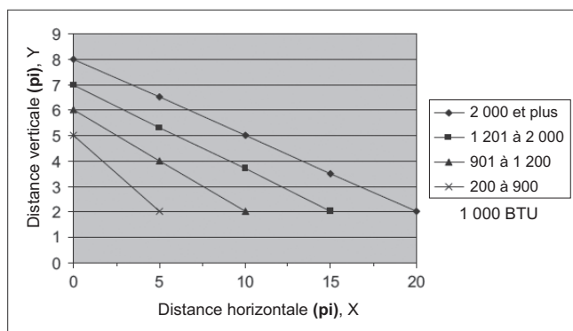
Figure 3 – Prise d'air et évacuation horizontales pour les systèmes à évacuation directe multiple
