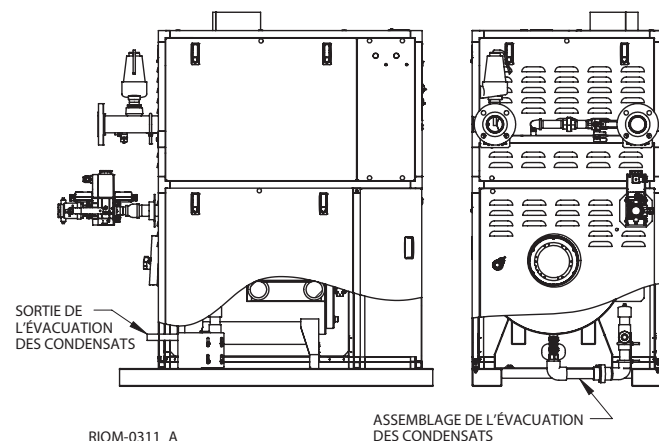
Figure 16 – Purgeur de condensats série Torus
