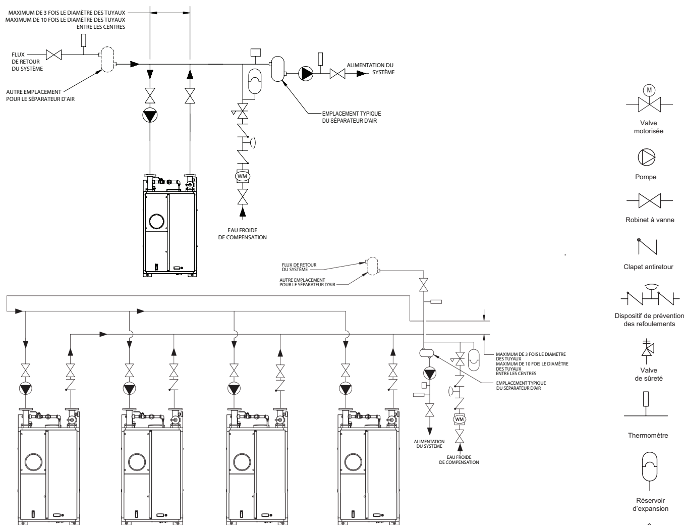
Figure 13 – Tuyauterie primaire/secondaire typique pour chaudière multiples – séparateur hydraulique (RECOMMANDÉ)
