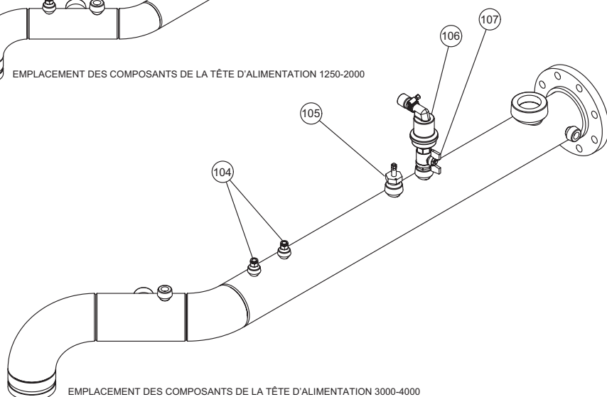
EMPLACEMENT DES COMPOSANTS DE LA TÊTE D'ALIMENTATION 3000-4000
