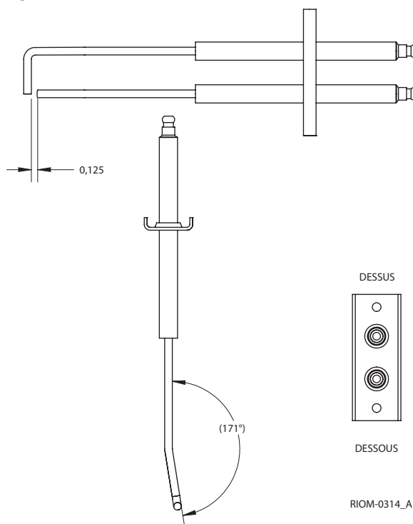
Figure 19a – Éclateur
