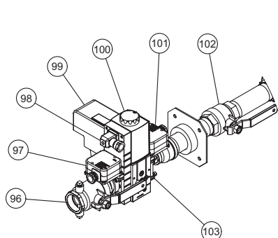
CIRCUIT DE VALVE À GAZ MBC 1000
