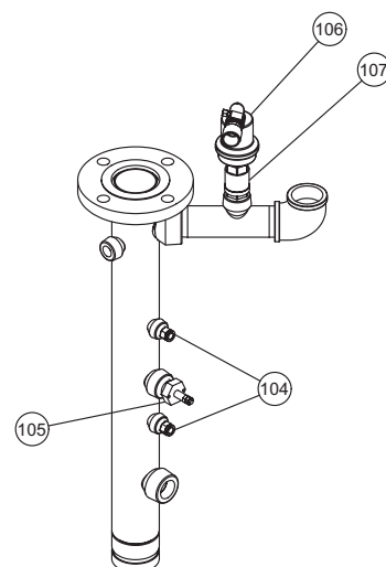
EMPLACEMENT DES COMPOSANTS DE LA TÊTE D'ALIMENTATION VERTICALE 1250-4000
