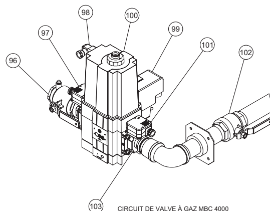
CIRCUIT DE VALVE À GAZ MBC 4000
