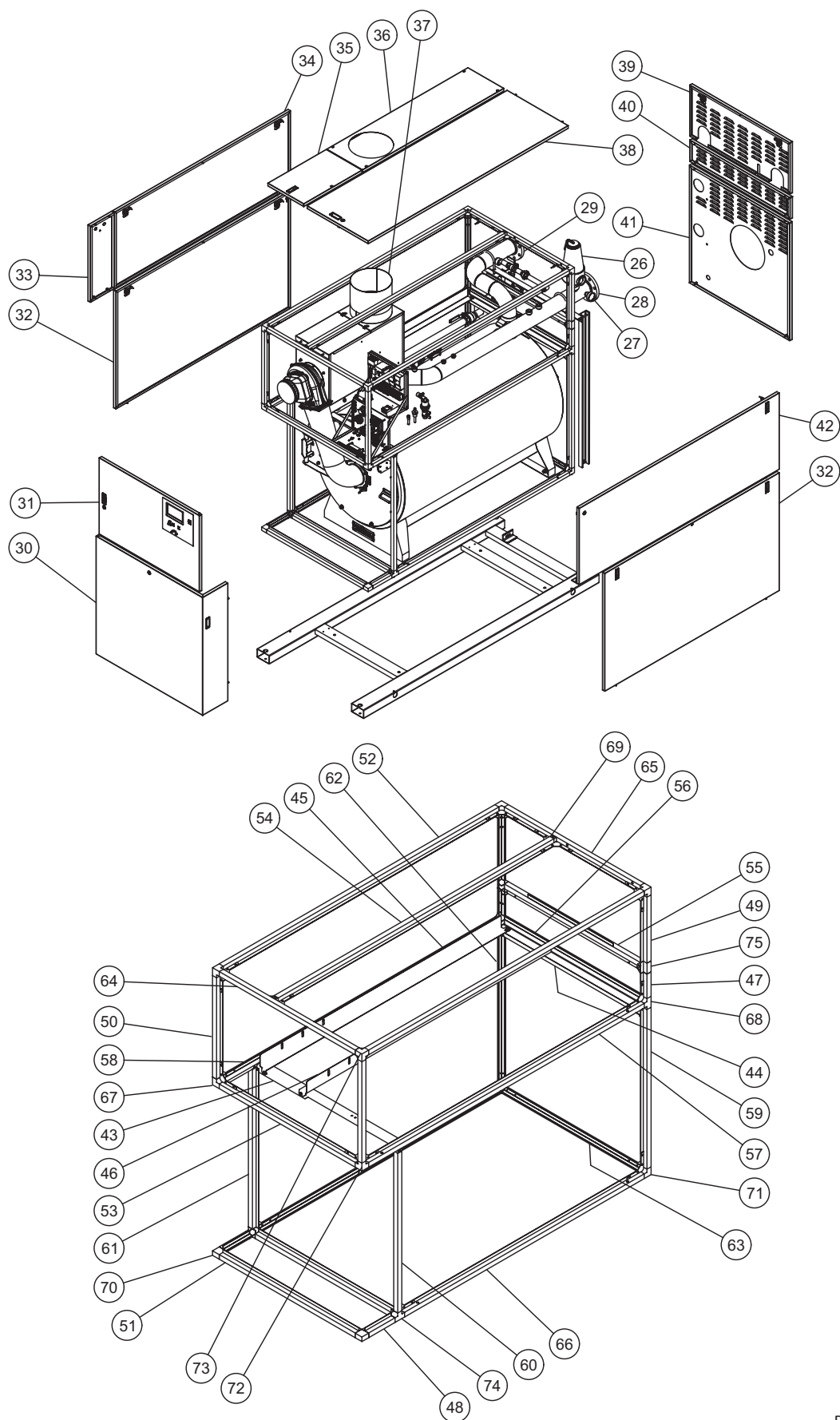
Figure 24 – Vue éclatée et pièces de rechange
