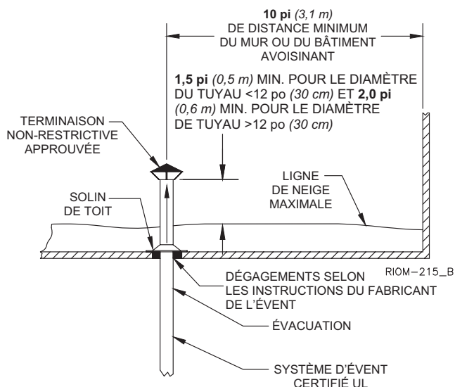
Figure 7 – Évent vertical à pression positive
