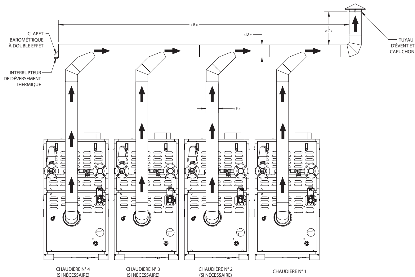
Figure 1 – Ventilation commune à plusieurs chaudières
