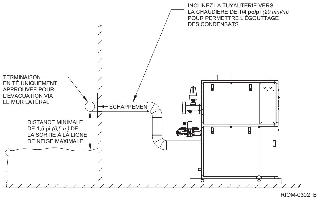
Figure 6 – Ventilation par la paroi latérale
