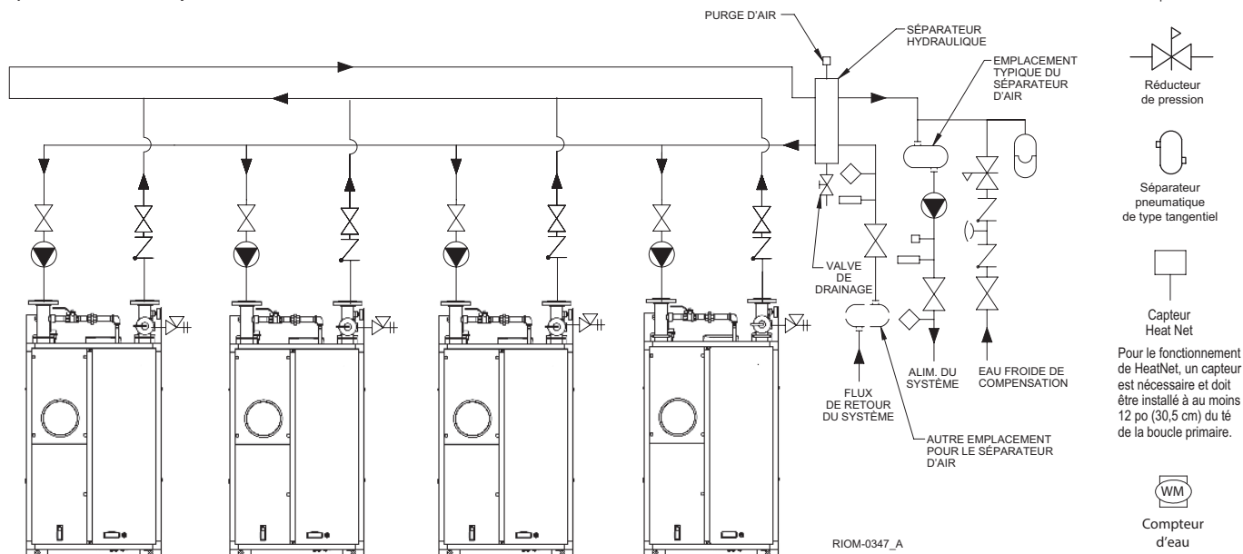
Figure 13 – Tuyauterie primaire/secondaire typique pour chaudière multiples – séparateur hydraulique (RECOMMANDÉ)
