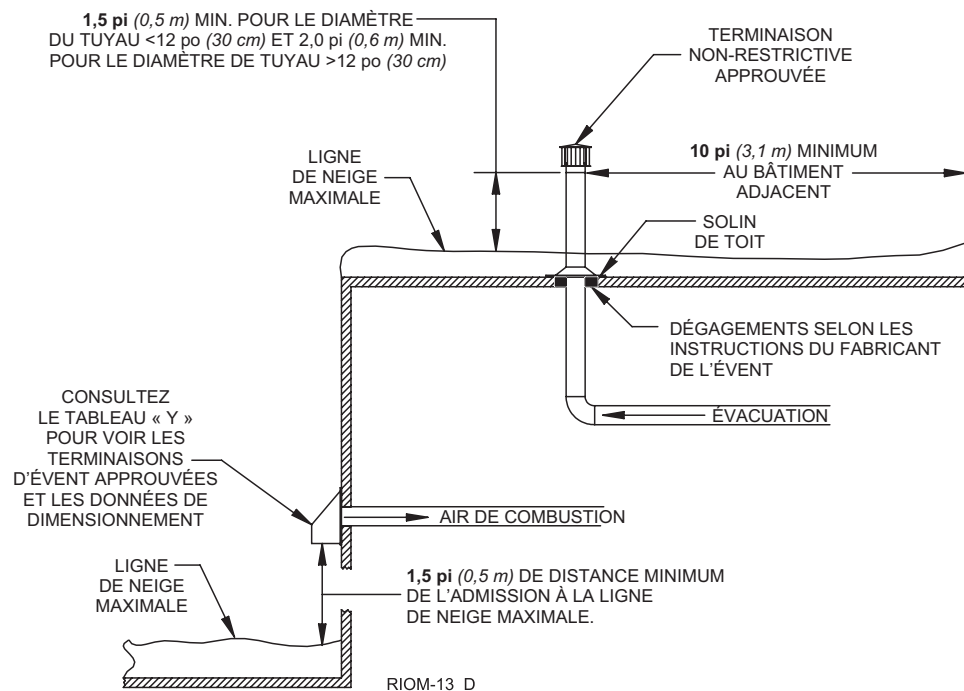
Figure 5 – Systèmes combinés à évacuation directe
