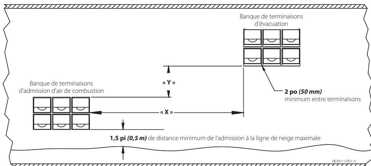
Figure 3 – Prise d'air et évacuation horizontales pour les systèmes à évacuation directe multiple
