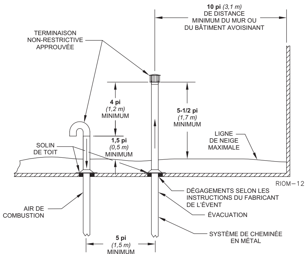
Figure 4 – Prise d'air et ventilation verticale pour système à évacuation directe
