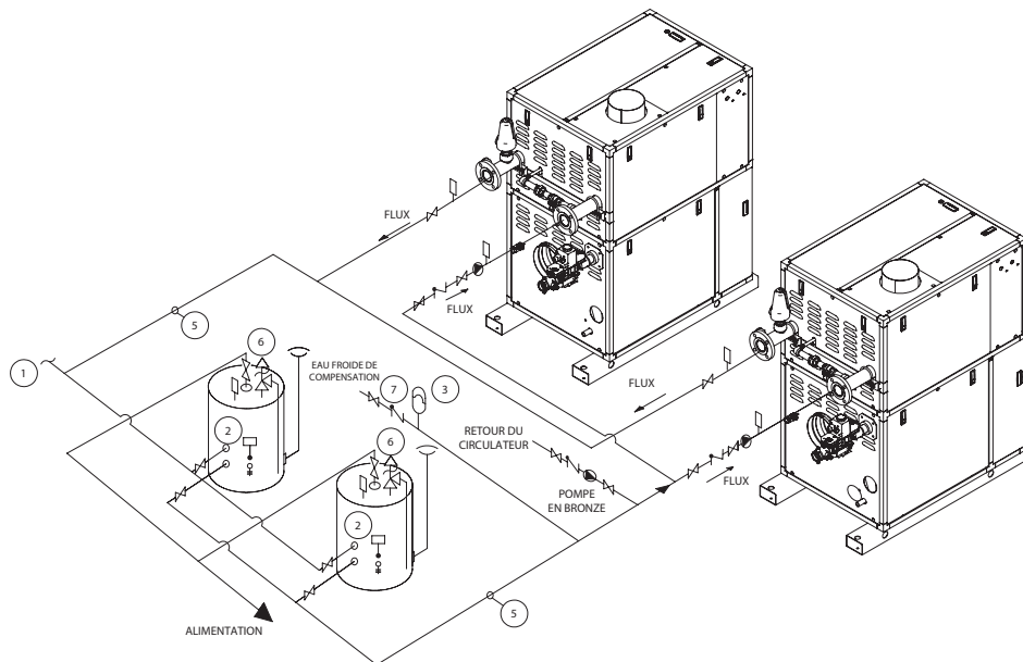
Figure 15 – Chaudière multiple typique avec tuyauterie de réservoir de stockage direct
