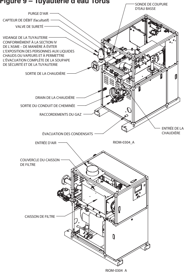
Figure 9 – Tuyauterie d'eau Torus
